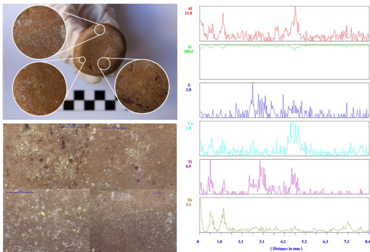
Figura 9. Fotografías de detalle y resultado de los análisis fisicoquímicos sobre el machacador de cuarcita.
