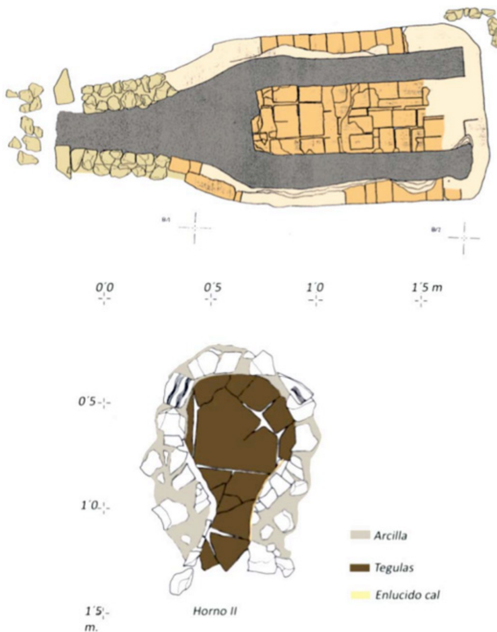
Figura 2. Planta de los hornos de la villa de Hellín documentados por García Blánquez. Fuente: Sanz Gamo, 2016: 163, Fig. 3.
